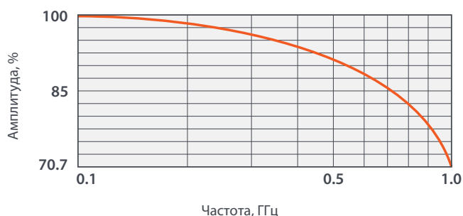
Рис. 1. Типовая амплитудно-частотная характеристика осциллографа общего назначения
