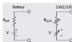
Упрощенная схема батареи и источника питания 2302/2306.
