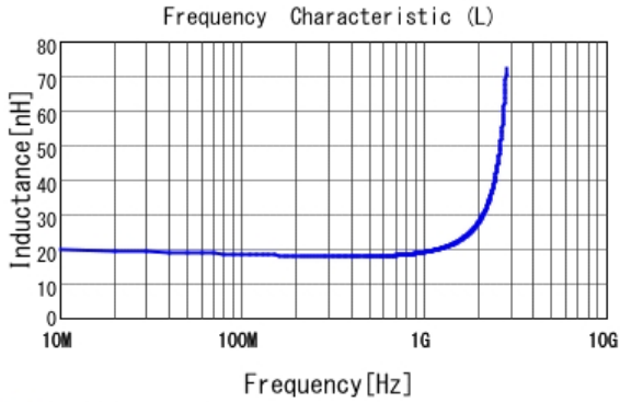
■ LQP03TN18NH02 L
