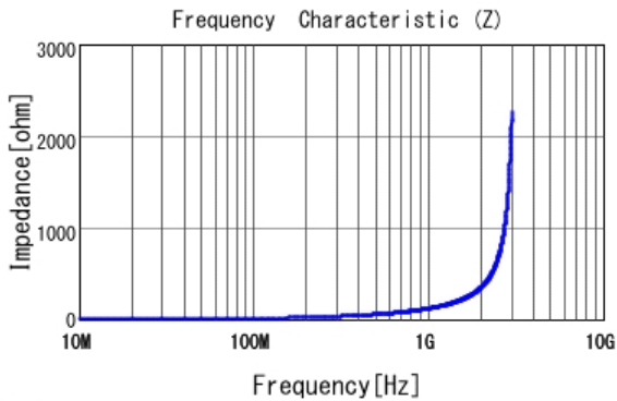
■ LQP03TN18NH02 |Z|
