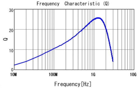
■ LQP03TN18NH02 Q
