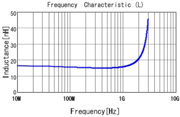
■ LQP03TN15NH02 L
