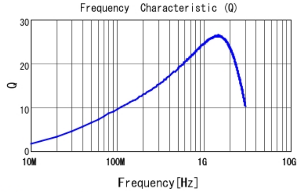
■ LQP03TN15NH02 Q
