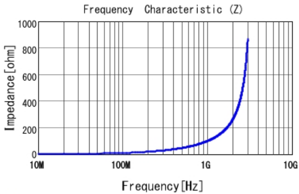
■ LQP03TN15NH02 |Z|
