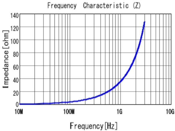
■ LQP03HQ5N6H02 |Z|
