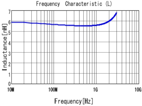
■ LQP03HQ5N6H02 L
