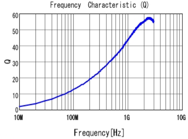
■ LQP03HQ5N6H02 Q
