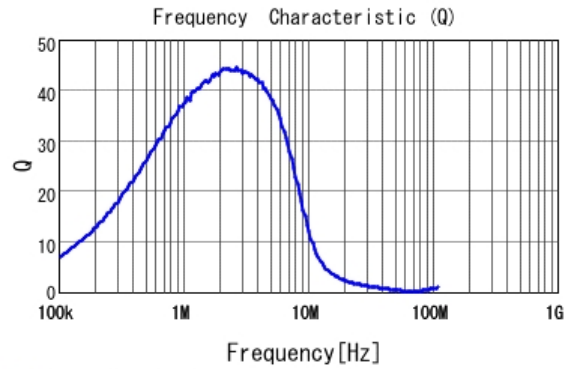
■ LQM18PN4R7MFR Q
