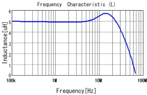
■ LQM18PN4R7MFR L
