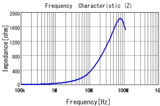
■ LQM18PN4R7MFR |Z|
