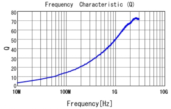
■ LQG18HN4N7S00 Q
