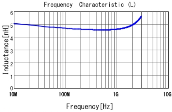
■ LQG18HN4N7S00 L
