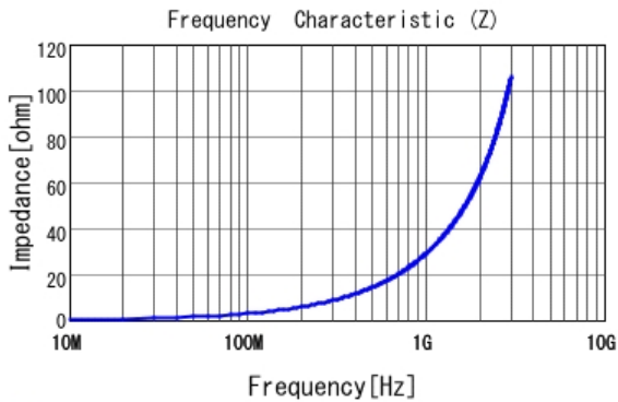
■ LQG18HN4N7S00 |Z|
