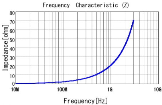
■ LQG18HN3N3S00 |Z|
