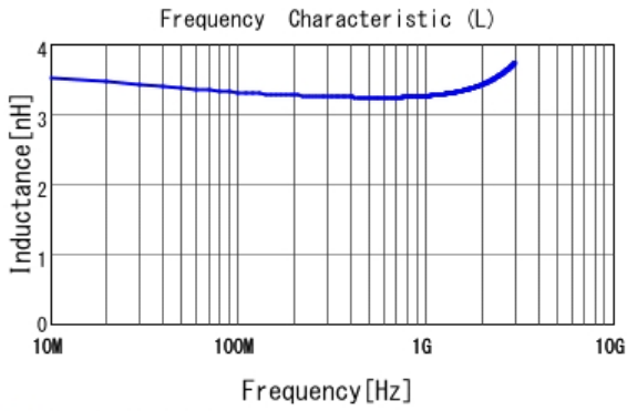
■ LQG18HN3N3S00 L
