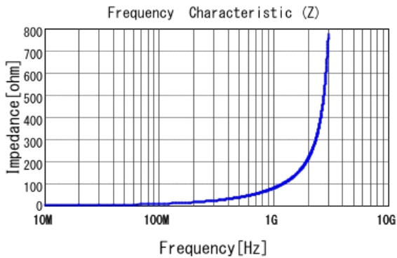
■ LQG18HN12NJ00 |Z|
