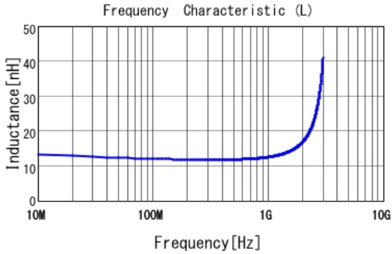
■ LQG18HN12NJ00 L
