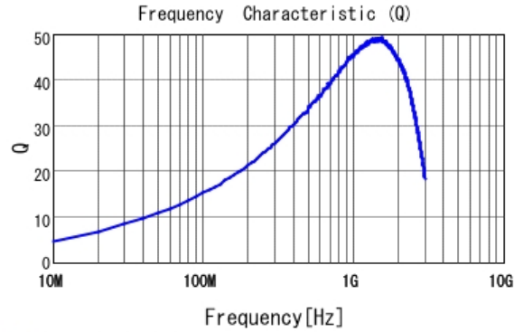
■ LQG18HN12NJ00 Q
