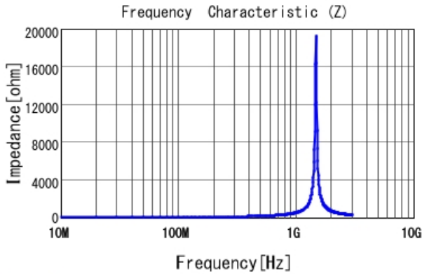
LQG18HH47NJ00 |Z|
