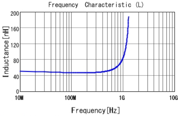
LQG18HH47NJ00 L
