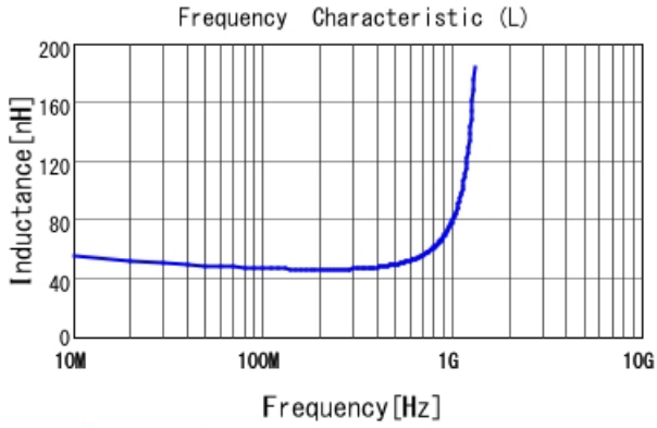
LQG15HZ47NJ02 L
