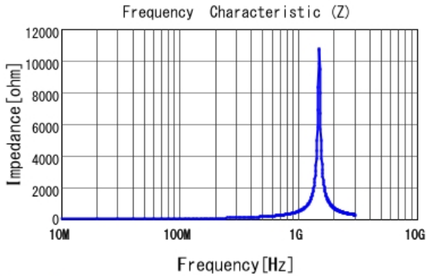
LQG15HZ47NJ02 |Z|
