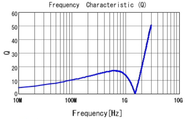
LQG15HZ47NJ02 Q
