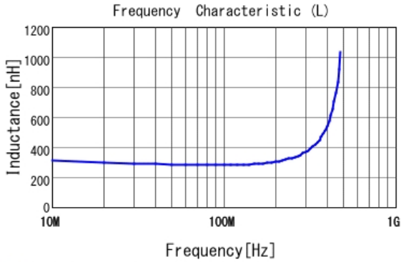
■ LQG15HSR27J02 L
