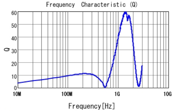
■ LQG15HSR27J02 Q
