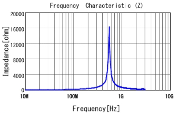
■ LQG15HSR27J02 |Z|
