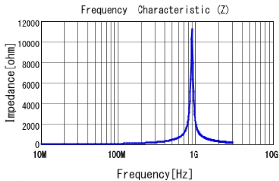
■ LQG15HSR10J02 |Z|
