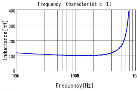
■ LQG15HSR10J02 L
