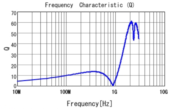
■ LQG15HSR10J02 Q
