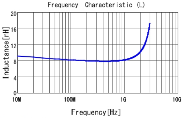
LQG15HS8N2H02 L
