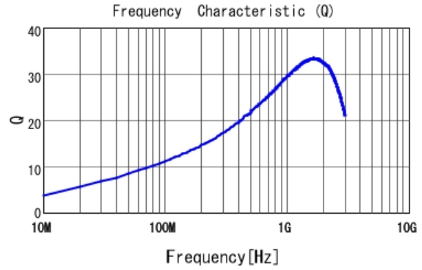
LQG15HS8N2H02 Q
