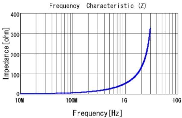
LQG15HS8N2H02 |Z|
