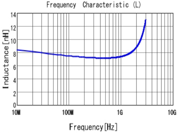
■ LQG15HS7N5H02 L
