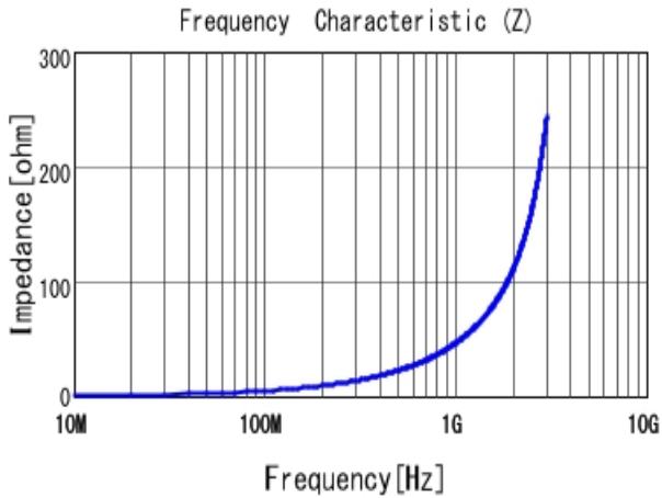
■ LQG15HS7N5H02 |Z|
