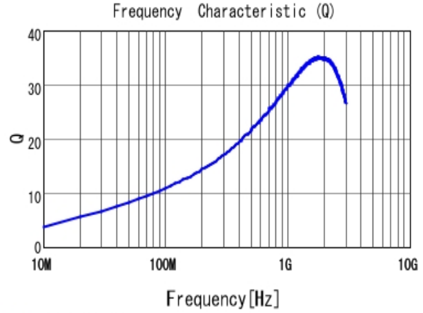
■ LQG15HS7N5H02 Q
