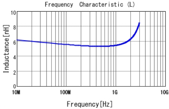
■ LQG15HS5N6S02 L
