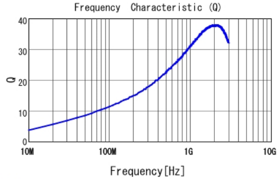
■ LQG15HS5N6S02 Q
