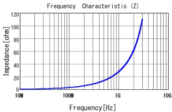
■ LQG15HS4N7S02 |Z|
