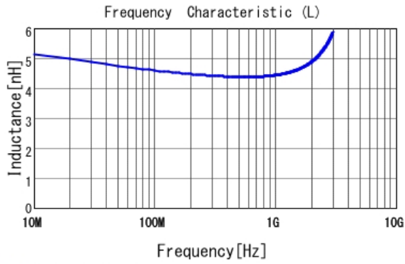
■ LQG15HS4N7S02 L
