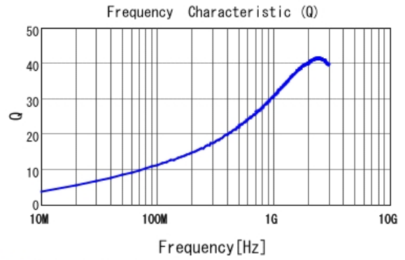
■ LQG15HS4N7S02 Q
