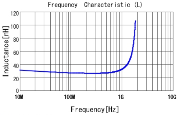
■ LQG15HS27NJ02 L
