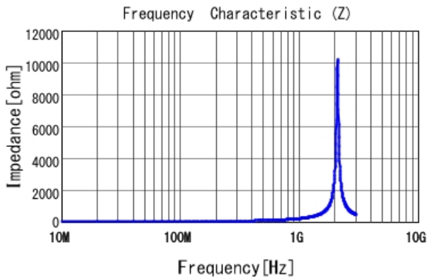
■ LQG15HS27NJ02 |Z|
