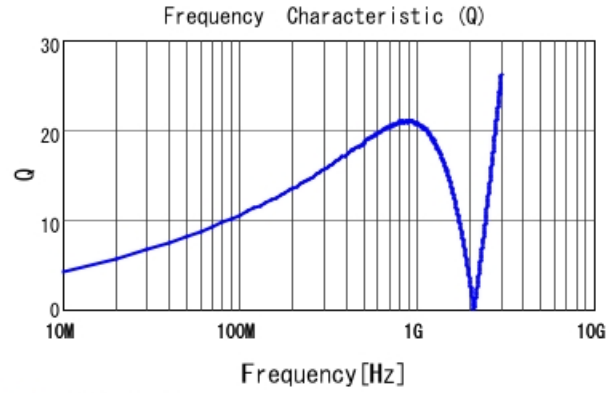
■ LQG15HS27NJ02 Q
