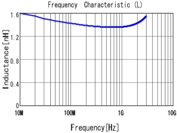
■ LQG15HS1N5S02 L
