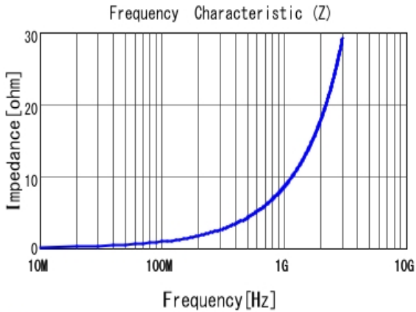
■ LQG15HS1N5S02 |Z|
