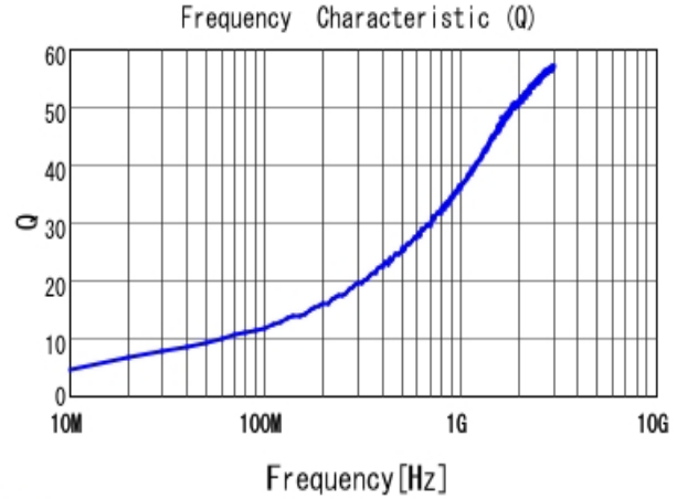
■ LQG15HS1N5S02 Q
