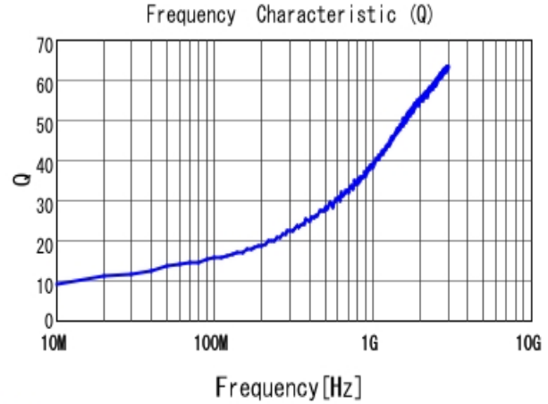
■ LQG15HS1N0C02 Q
