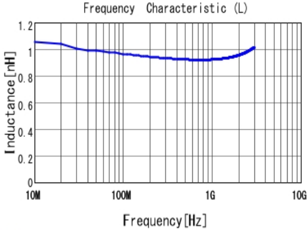
■ LQG15HS1N0C02 L
