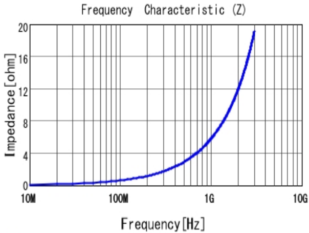
■ LQG15HS1N0C02 |Z|
