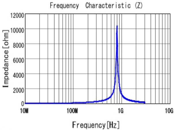
■ LQG15HNR12J02 |Z|
