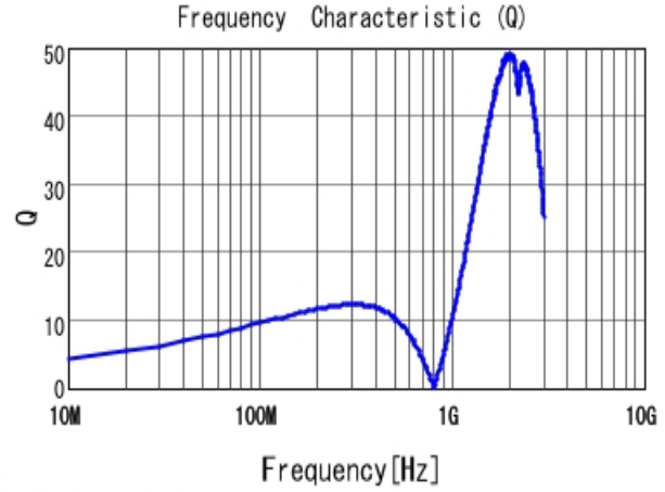
■ LQG15HNR12J02 Q
