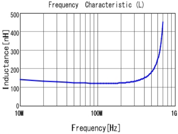
■ LQG15HNR12J02 L
