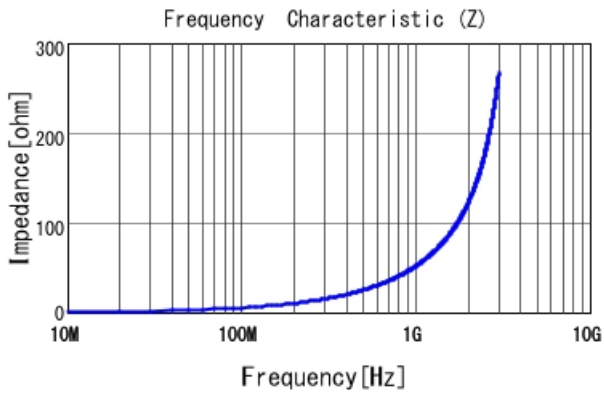
■ LQG15HN8N2J02 |Z|
