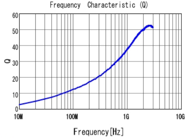
■ LQG15HN3N9S02 Q
