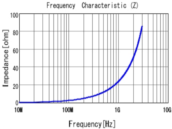
■ LQG15HN3N9S02 |Z|
