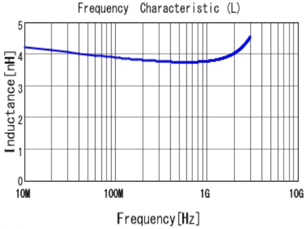
■ LQG15HN3N9S02 L
