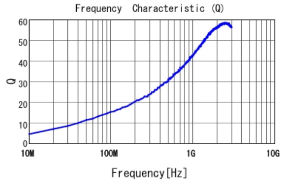
■ LQG15HN2N7S02 Q
