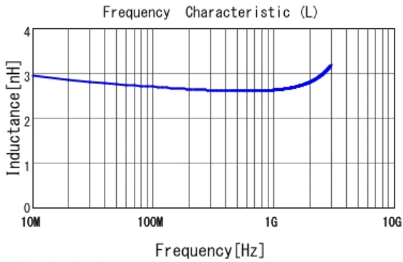
■ LQG15HN2N7S02 L
