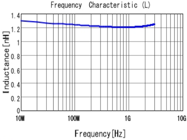
■ LQG15HN1N2S02 L
