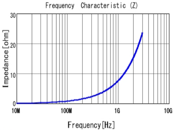
■ LQG15HN1N2S02 |Z|
