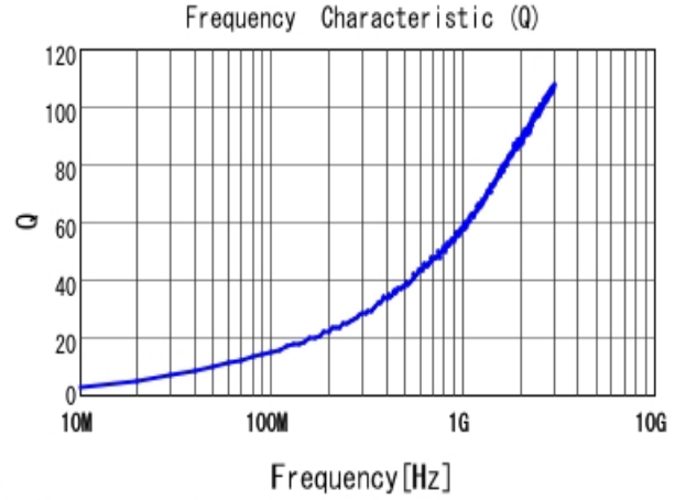
■ LQG15HN1N2S02 Q
