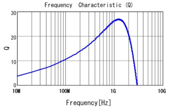
■ LQG15HN15NJ02 Q
