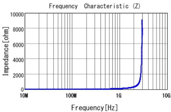
■ LQG15HN15NJ02 |Z|
