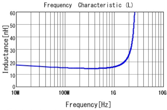
■ LQG15HN15NJ02 L
