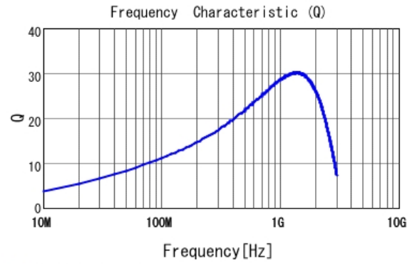
■ LQG15HN12NJ02 Q
