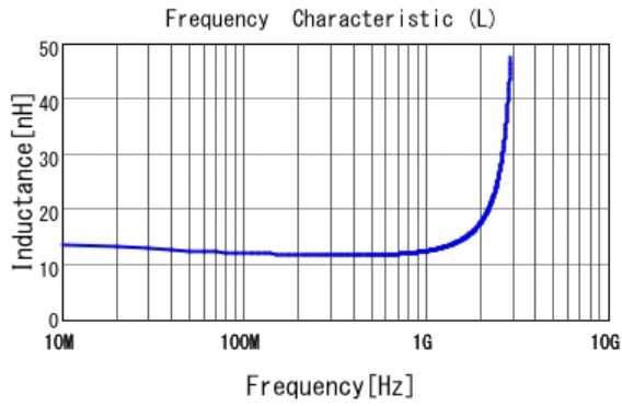
■ LQG15HN12NJ02 L
