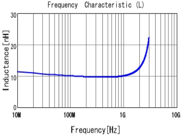
■ LQG15HH10NJ02 L
