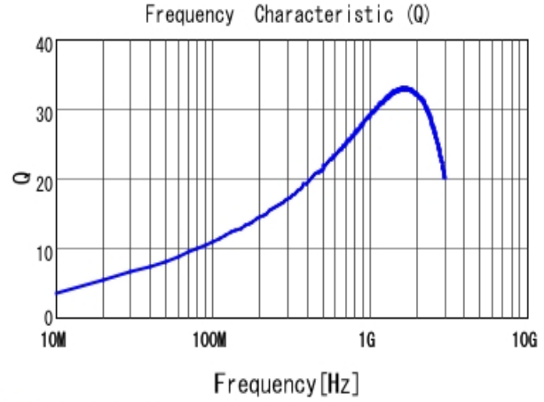
■ LQG15HH10NJ02 Q
