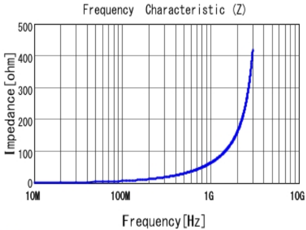
■ LQG15HH10NJ02 |Z|
