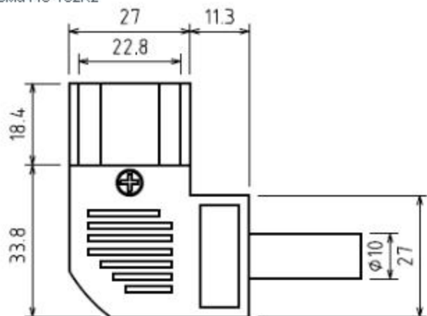
Схема AC-102R2
