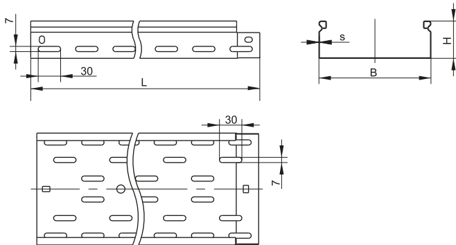
Рисунок 1. Габаритные размеры лотка перфорированного серии ESCA
