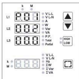
Esempio impostazione rapporto TA: TA 1000/5A settare P01=200. Example of CT ratio programming: with 1000/5A CT, set P01 to 200. Exemple de réglage rapport TI : avec TI 1000/5A, réglez P01 à 200. Ejemplo de programación de relación de TC: Con un TC de 1000/5A, ajustar P01 a 200.
