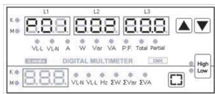
Esempio impostazione rapporto TA: TA 1000/5A settare P01=200. Example of CT ratio programming: with 1000/5A CT, set P01 to 200. Exemple de réglage rapport TI : avec TI 1000/5A, réglez P01 à 200. Ejemplo de programación de relación de TC: Con un TC de 1000/5A, ajustar P01 a 200.
