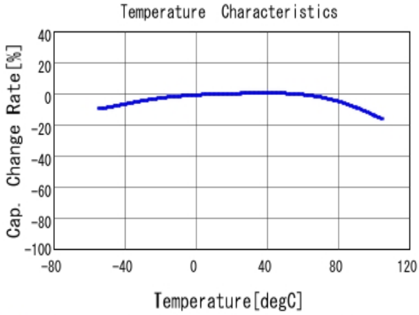
■ LLL153C80J224ME14 C-Temp. capchange, DCO. 0V, ACO. 5V rm
