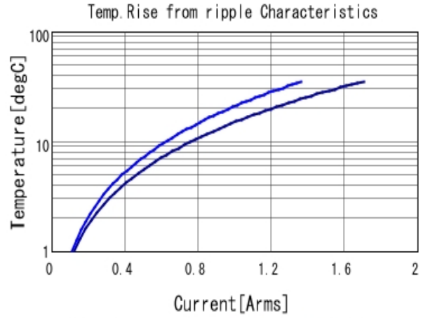
LLL153C80J224ME14 Temp. rise ■ 500kHz ■ 1MHz
