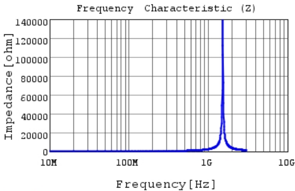
LQW18ANR22G00 |Z|
