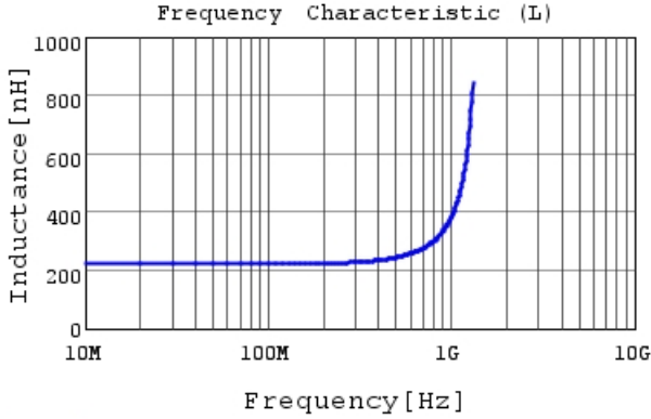
LQW18ANR22G00 L
