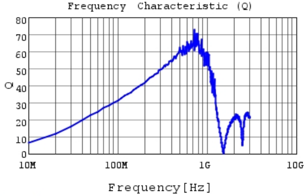
LQW18ANR22G00 Q
