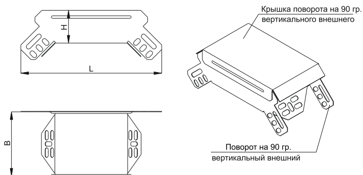
Рисунок 1. Габаритные размеры поворота на 90град вертикального внешнего серии ESCA
