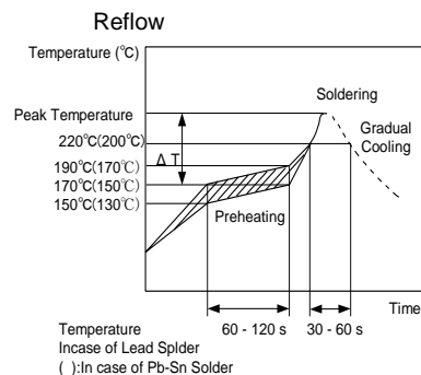
Vapor Reflow
