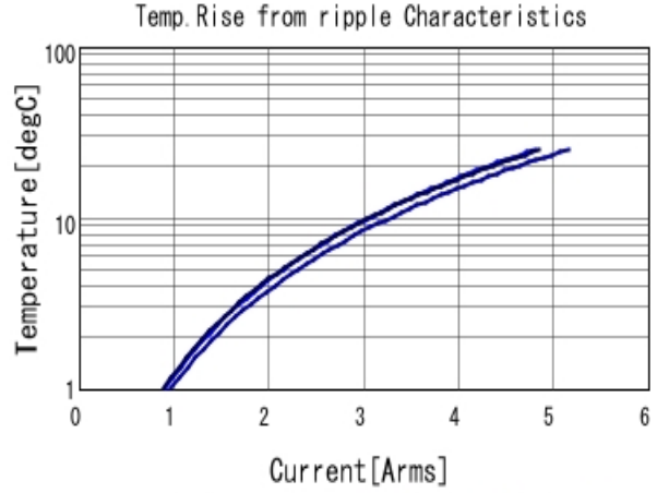
KCM55WR7YA476MH01 Temp. rise ■ 50kHz ■ 100kHz ■ 300kHz
