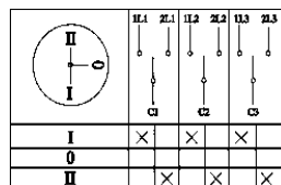
Пакетный переключатель ППП 3-полюсный на 2 направления
