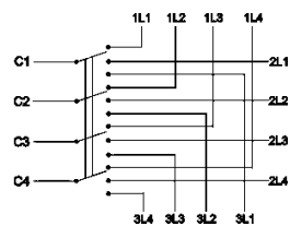
Пакетный переключатель ППП 4-полюсный на 3 направления
