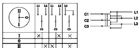
Пакетный переключатель ПП 3-полюсный реверсный
