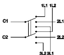
Пакетный переключатель ППП 2-полюсный на 3 направления
