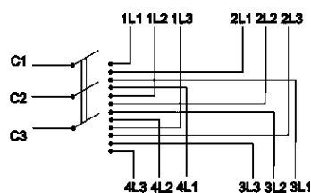
Пакетный переключатель ППП 3-полюсный на 4 направления
