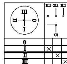
Пакетный переключатель ППП 1-полюсный на 3 направления
