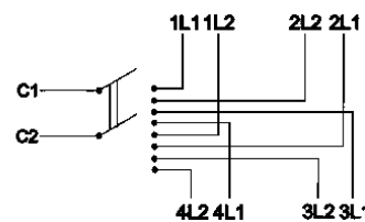
Пакетный переключатель ППП 2-полюсный на 4 направления
