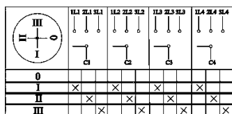
Пакетный переключатель ППП 4-полюсный на 3 направления
