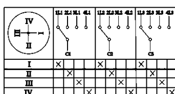
Пакетный переключатель ППП 3-полюсный на 4 направления
