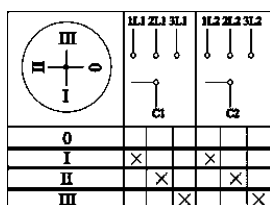
Пакетный переключатель ППП 2-полюсный на 3 направления
