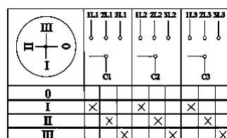
Пакетный переключатель ППП 3-полюсный на 3 направления
