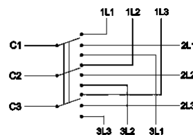
Пакетный переключатель ППП 3-полюсный на 3 направления
