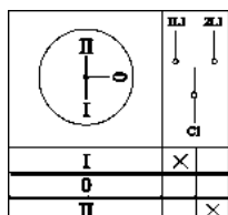
Пакетный переключатель ППП 1-полюсный на 2 направления
