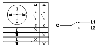
Пакетный переключатель ПП 1-полюсный 4C специального исполнения
