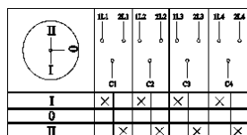
Пакетный переключатель ППП 4-полюсный на 2 направления
