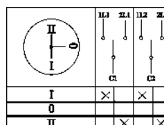
Пакетный переключатель ППП 2-полюсный на 2 направления
