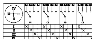
Пакетный переключатель ППП 4-полюсный на 4 направления
