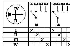
Пакетный переключатель ППП 2-полюсный на 4 направления
