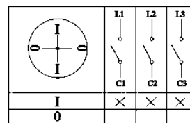
Пакетный выключатель ПВ 3-полюсный
