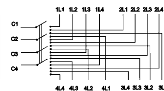
Пакетный переключатель ППП 4-полюсный на 4 направления
