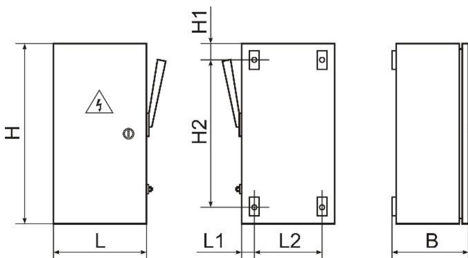
Рисунок 1. Общий вид и габаритные размеры ящиков силовых
