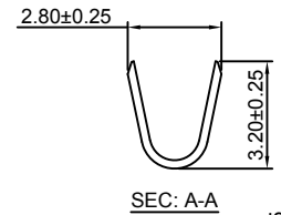
SEC: A-A
