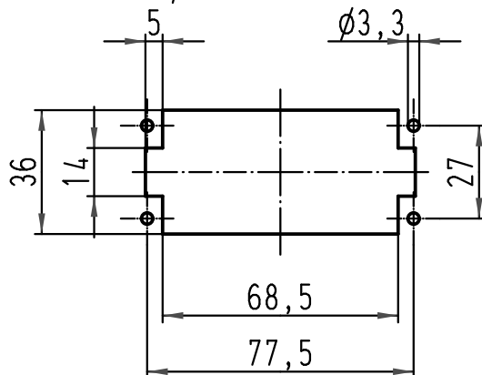
1:2 Montageausschnitt panel cut out
