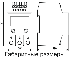
Габаритные размеры
