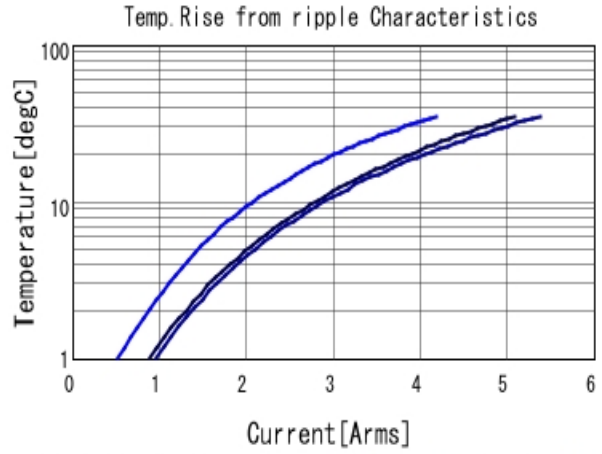
■ GRT31CR61H106KE01 Temp. rise ■ 100kHz ■ 500kHz ■ 1MHz
