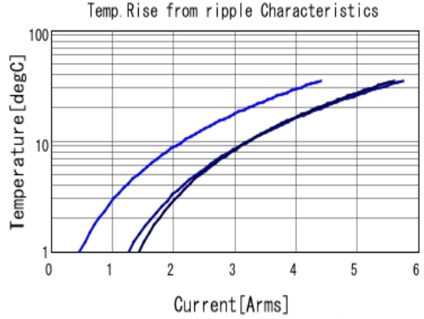
■ GRT21BR61A226ME13 Temp. rise ■ 80kHz ■ 400kHz ■ 800kHz
