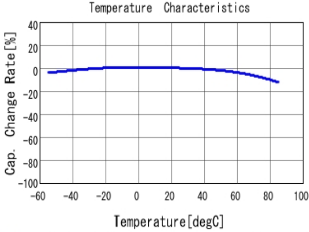
■ GRT21BR61A226ME13 C-Temp. capchange, DCO. 0V, ACO. 5Vrm
