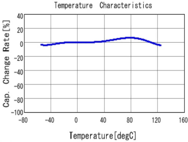
■ GRT155R70J105KE01 C-Temp. capchange, DCO. 0V, ACO. 5V rm
