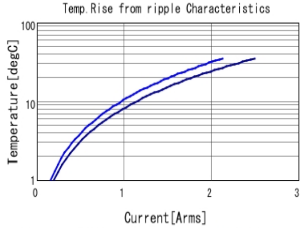
■ GRT155R70J105KE01 Temp. rise ■ 500kHz ■ 1MHz
