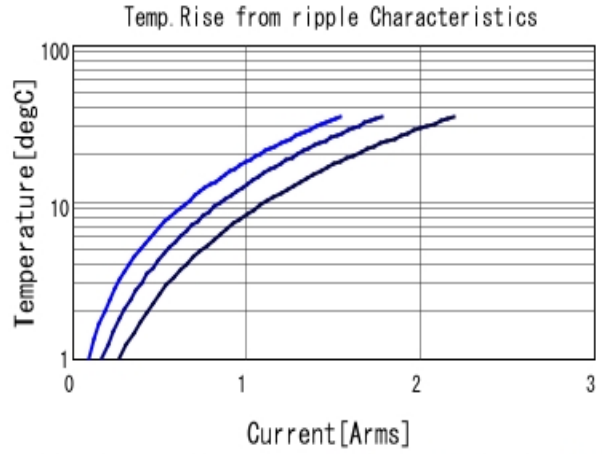
■ GRT155R6YA474KE01 Temp. rise ■ 200kHz ■ 500kHz ■ 1MHz
