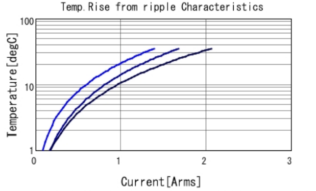
GRT155R61E474KE01 Temp. rise — 200kHz — 500
