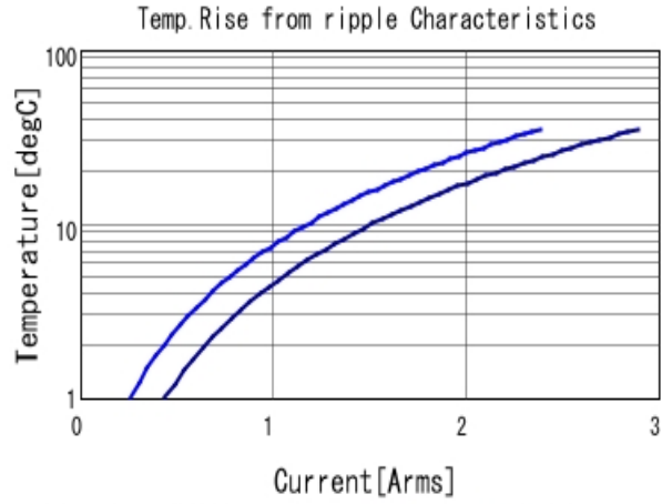
■ GRT155R61E105KE01 Temp. rise ■ 500kHz ■ 1MHz
