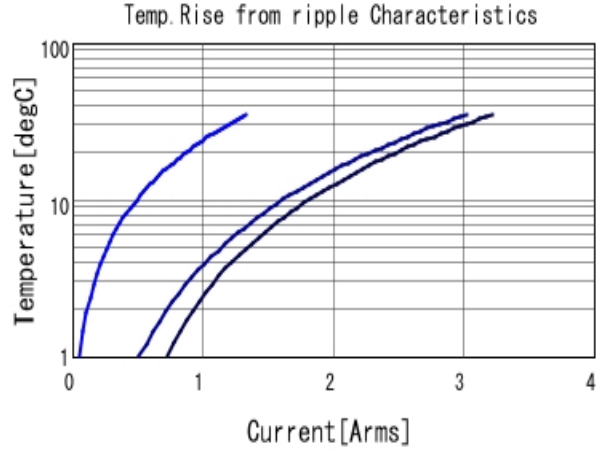
GRT155R61C474KE01 Temp. rise ■ 200kHz ■ 500kHz ■ 1MHz
