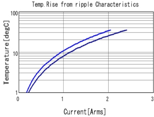
■ GRT155R61C105KE01 Temp. rise ■ 500kHz ■ 1MHz
