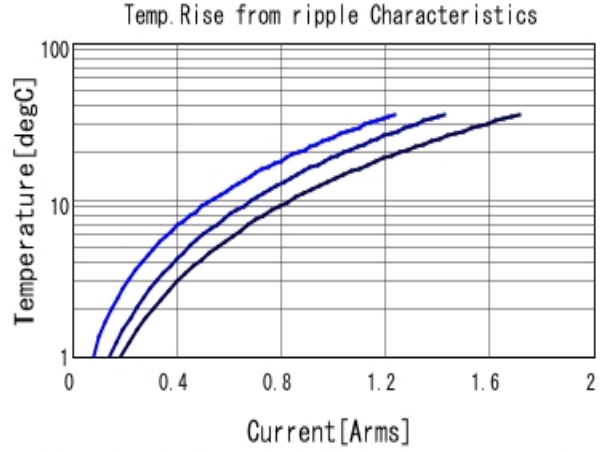
GRT155C8YA224KE01 Temp. rise ■ 300kHz ■ 600kHz ■ 1MHz
